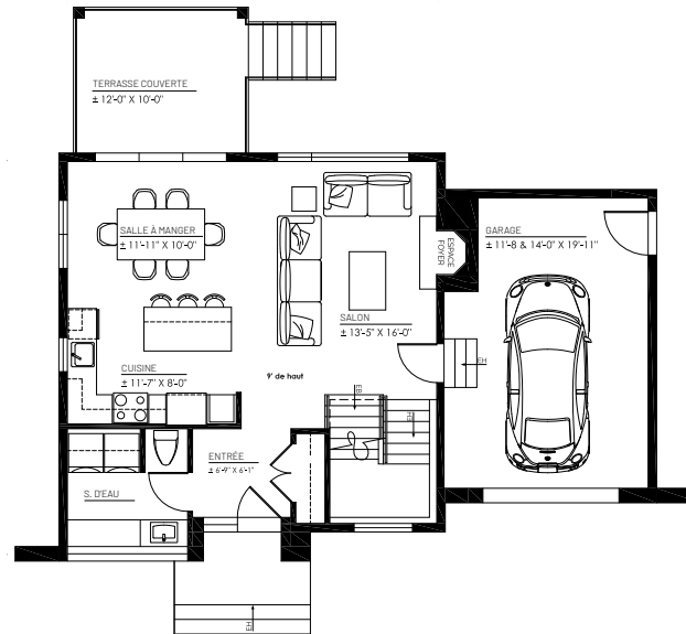
Rez-de-chaussée
